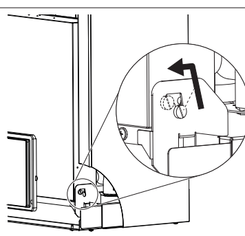
fig. 18 - come sbloccare la scatola elettrica
