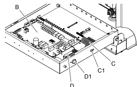
fig. 20 - vista interna del quadro elettrico
