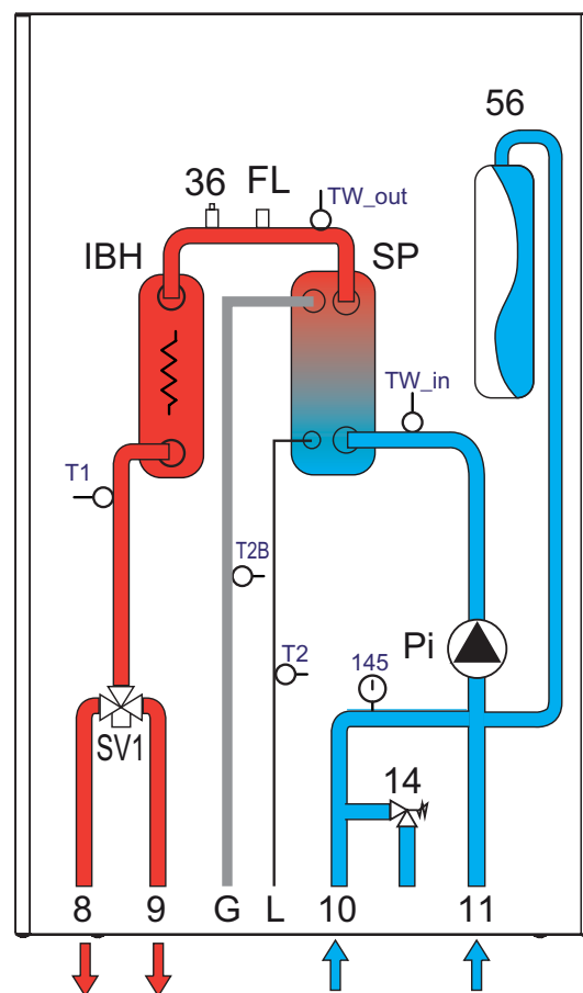
fig. 5 - Schema idraulico unità interna
