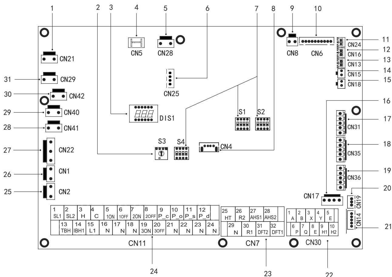
fig. 21 - Scheda idronica
