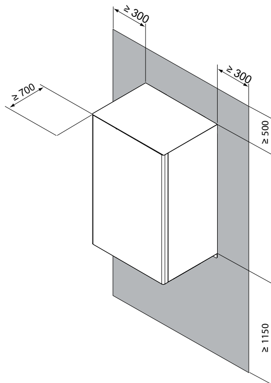
fig. 7 - area operativa minima per l'unità interna
